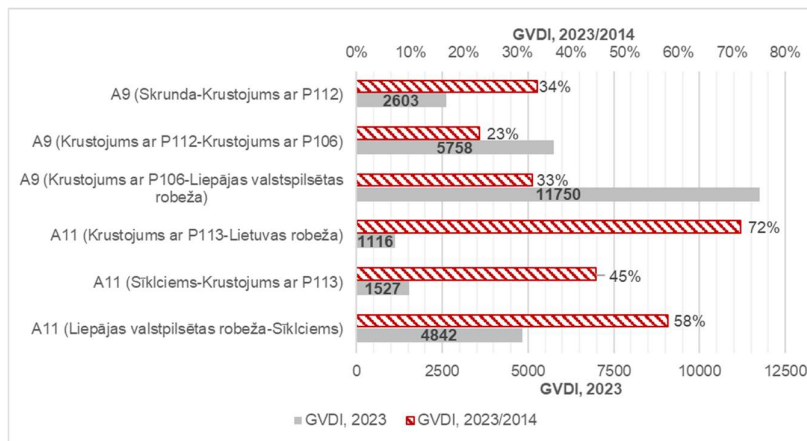
2-19. ATTĒLS. VIEGLO AUTOMOBILU GVDS VALSTS GALVENO AUTOCEĻU A9 UN A11 DIENVIDKURZEMES NOVADA POSMOS, 2023.(2014) G.
