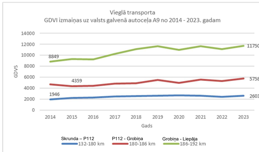
2-20. ATTĒLS. VIEGLĀ AUTOTRANSPORTA GADA VIDĒJĀS DIENNAKTS SATIKSMES IZMAINAS UZ VALSTS GALVENĀ AUTOCEĻA A9 “RĪGA (SKULTE) - LIEPĀJA” LAIKA POSMĀ NO 2014. LĪDZ 2023. G.
