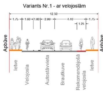
4-33. ATTĒLS. VARIANTS NR.1 AR VELOJOSLĀM
