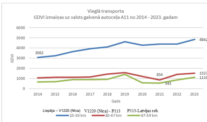
2-21. ATTĒLS. VIEGLĀ AUTOTRANSporta GADA VIDĒJĀS DIENNAKTS SATIKSMES IZMAIŅAS UZ VALSTS GALVENĀ AUTOCEĻA A11 “LIEPĀJA – LIETUVAS ROBEŽA (RUCAVA)” LAIKA POSMĀ NO 2014. LĪDZ 2023. G.
